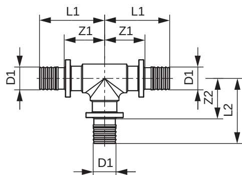
Тройник TECEflex
