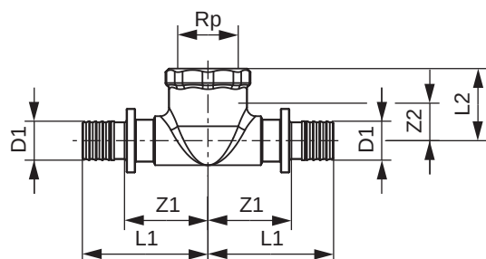
Тройник TECEflex, с внутренней резьбой
